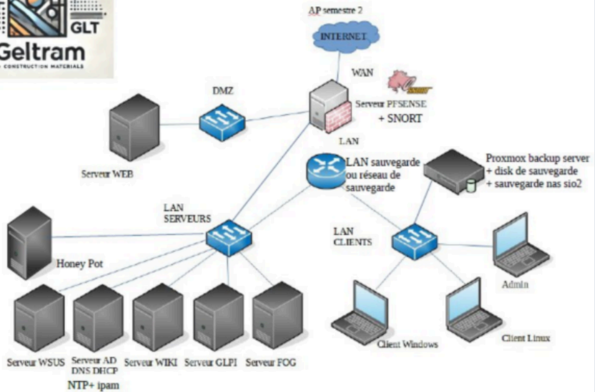
SCHEMA GELTRAM
